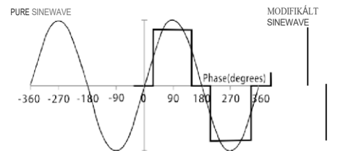
Módosított szinuszhullám és tiszta szinuszhullám összehasonlítása
